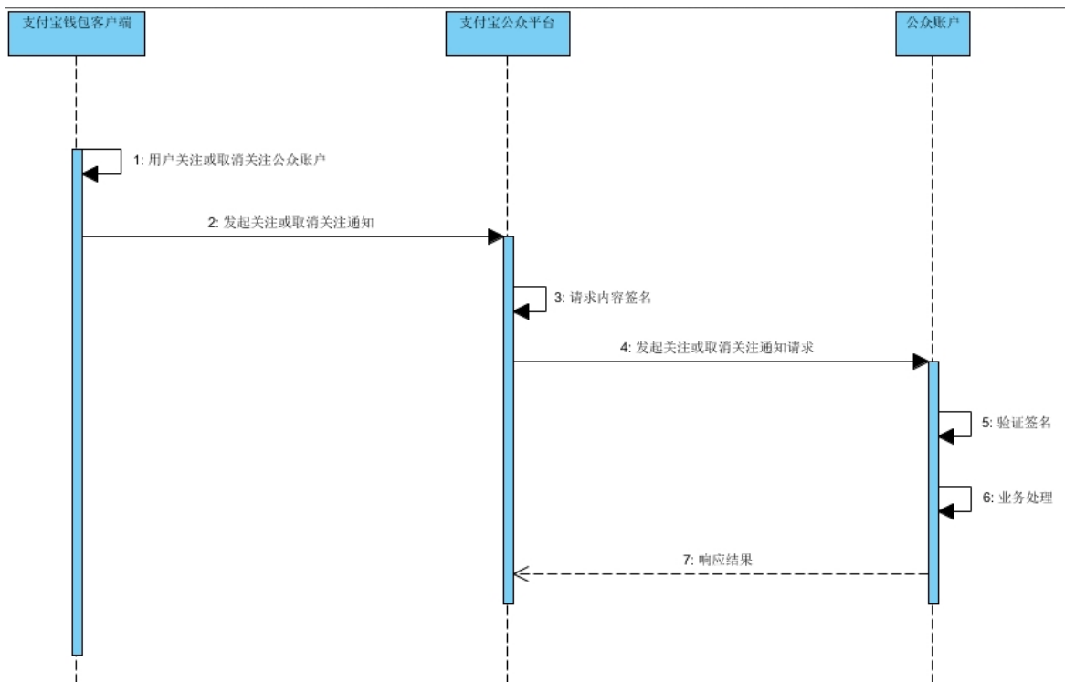
图2-1 接收关注或取消关注通知流程
