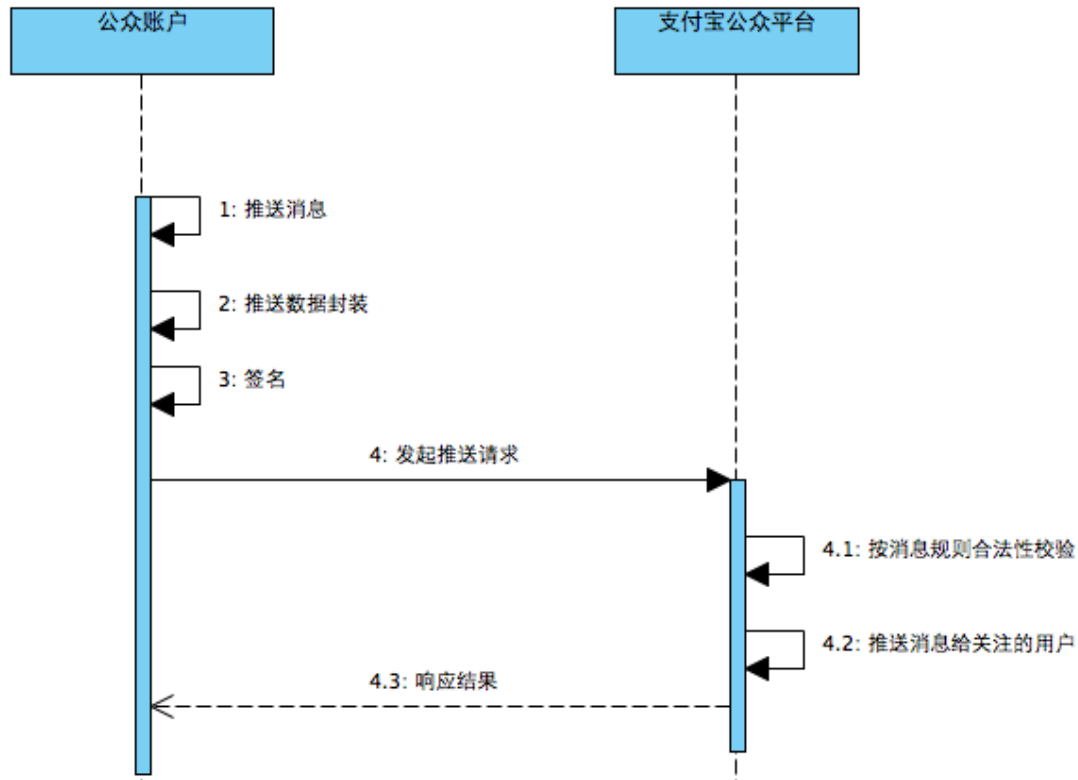
图2-3 公众账号推送消息流程
