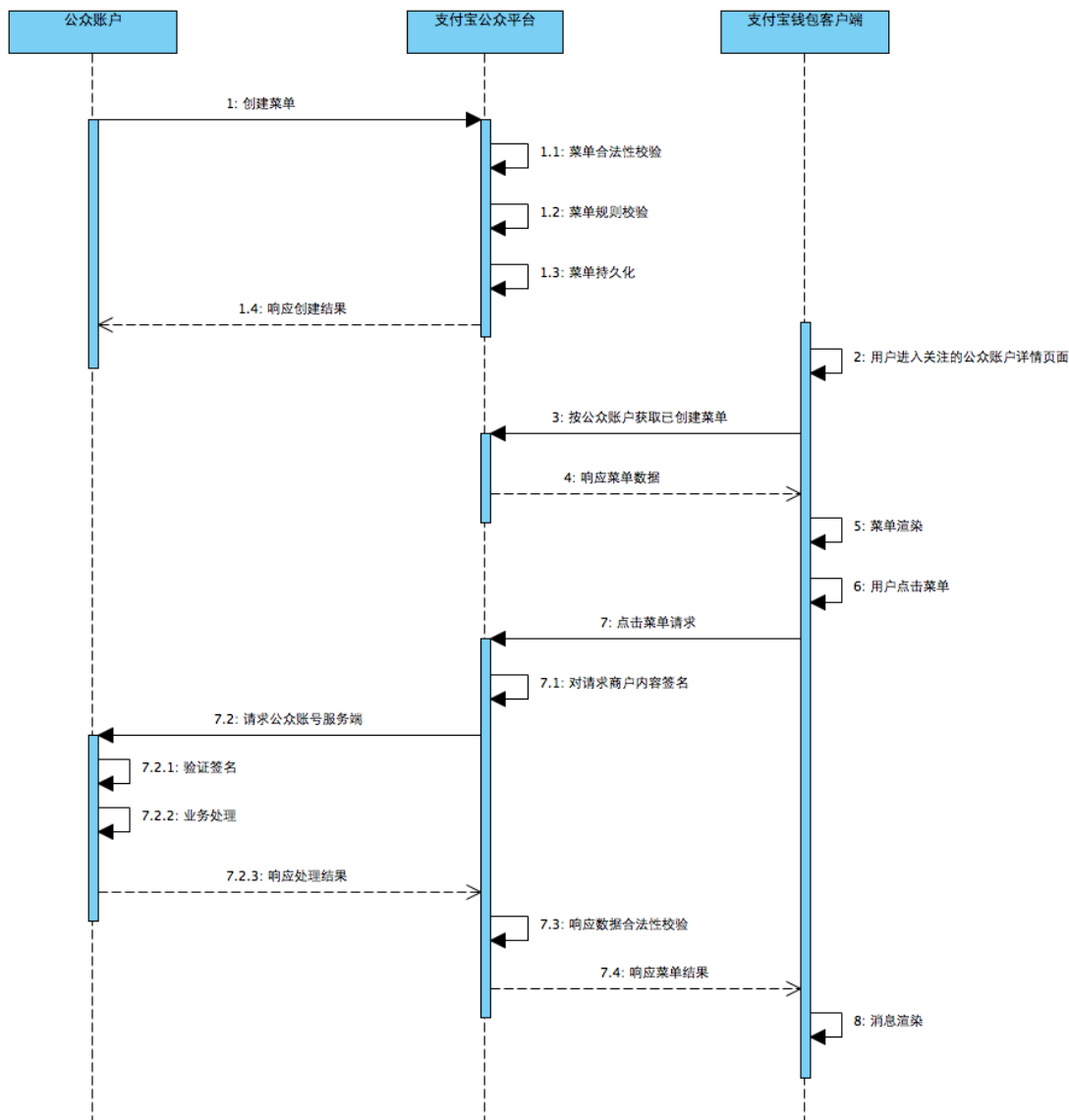
图2-2 公众账号菜单设置及响应流程
