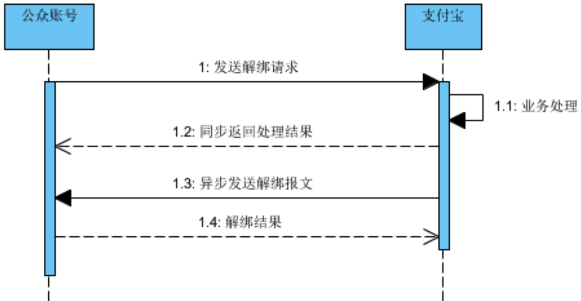
图2-5 发送解除绑定商户会员号成功通知流程
