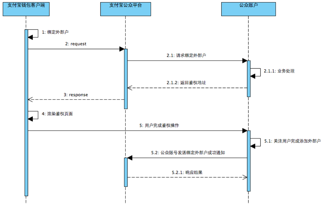
图2-4 公众账号发送绑定商户会员号成功通知流程
